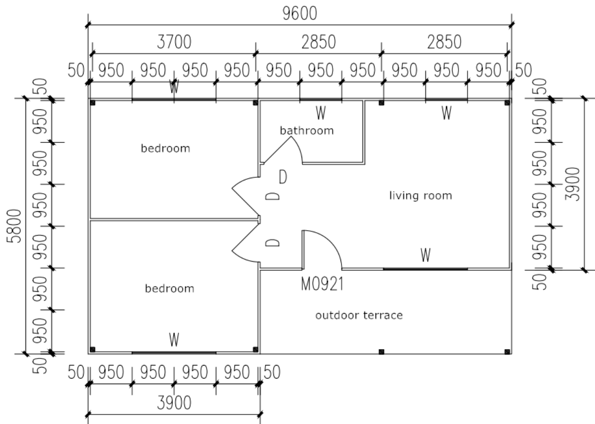
Beispielgrundriss ca. 55m 2
